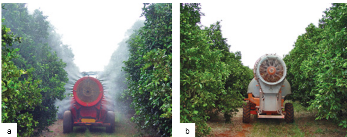
Figura 14 – Turbina muito baixa para a cultura (a), turbina na altura adequada (b).
