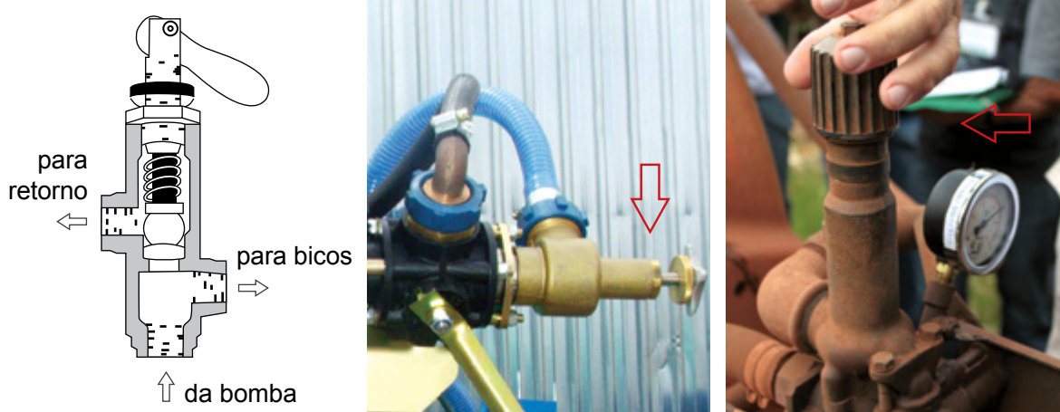
Figura 7 – Regulador de pressão 1.
