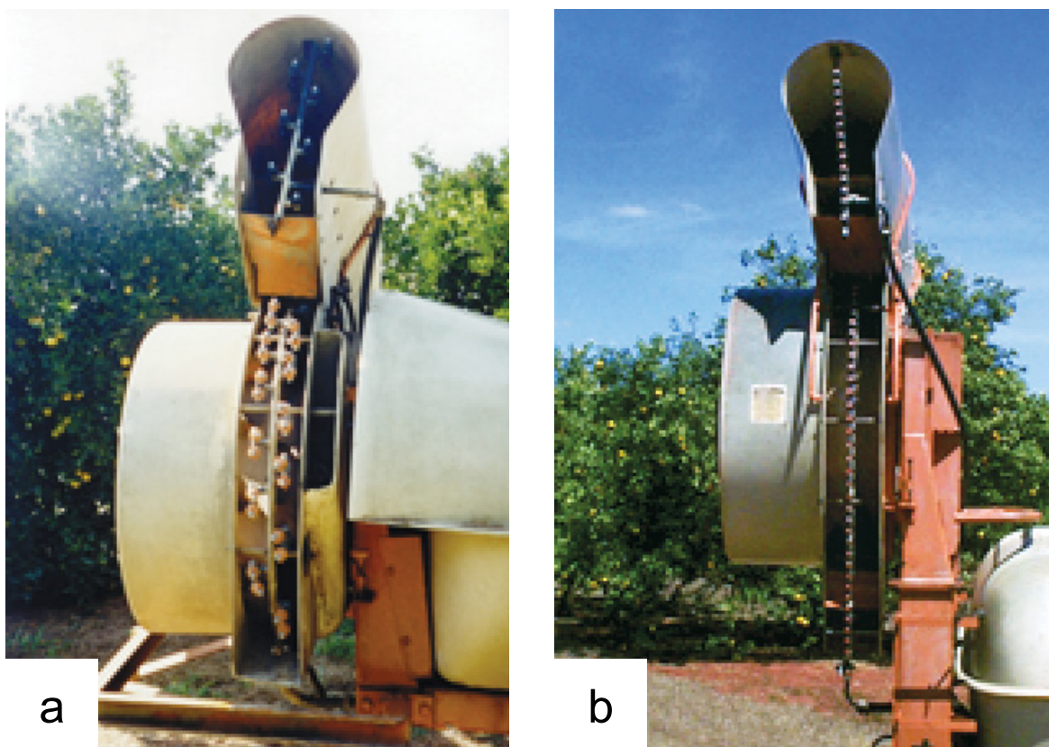
Figura 15 – Aumento do número de bicos na barra por meio do uso de duplicadores (a) ou pela utilização de barra com maior número de bicos (b).
