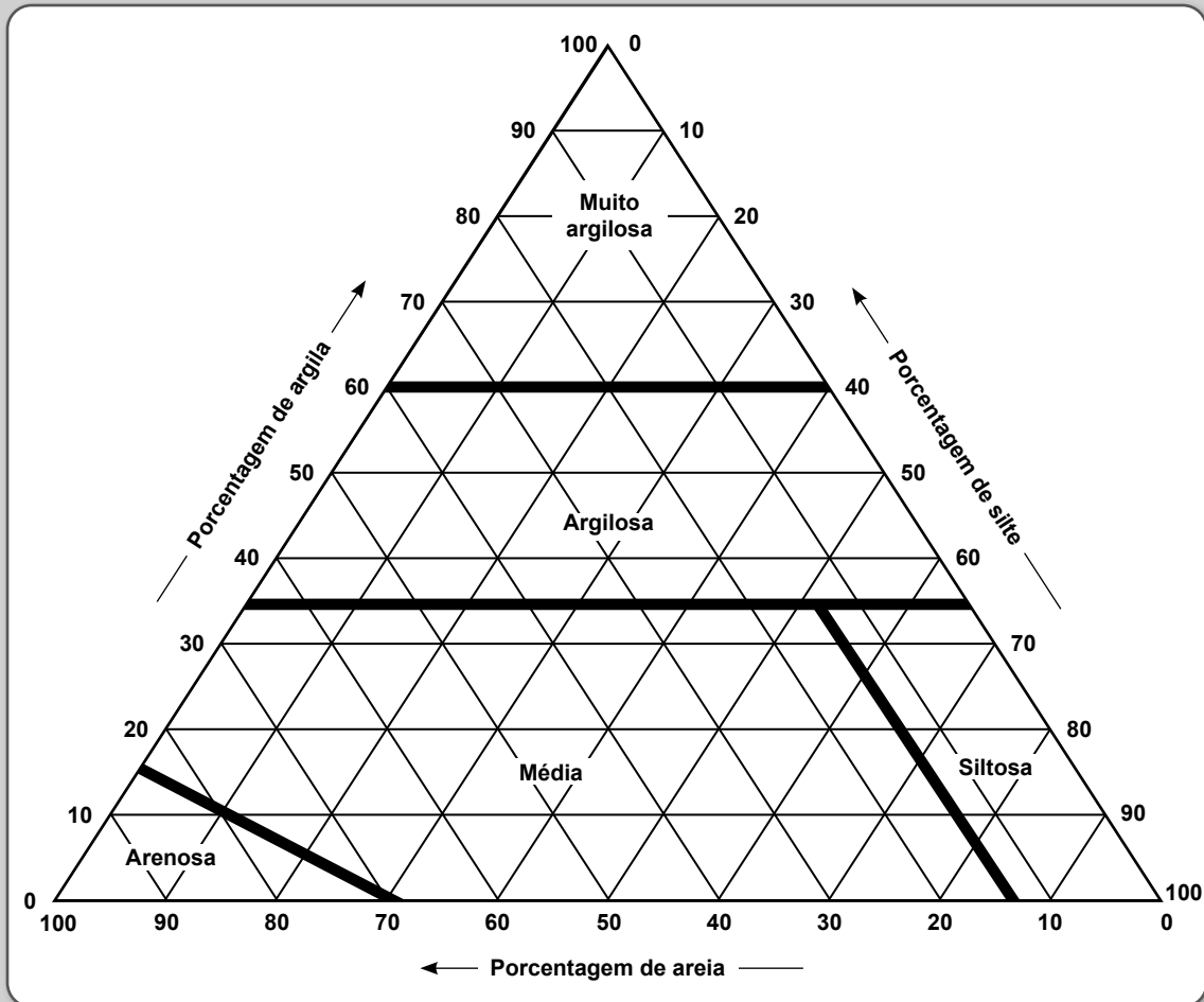
Figura 15 – Triângulo de grupamento textural.
