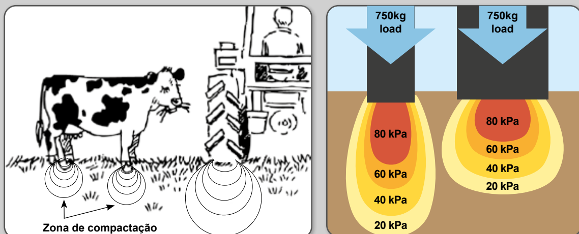
Figura 62 – Áreas de compactação por tráfego de máquinas e animais, e devido à largura da tala do pneu.
