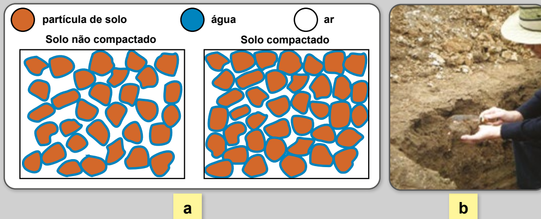
Figura 21 – Esquema da porosidade do solo (a) e verificação no campo (b).
