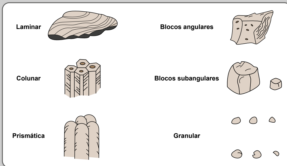
Figura 17 – Tipos de Estrutura do Solo.
