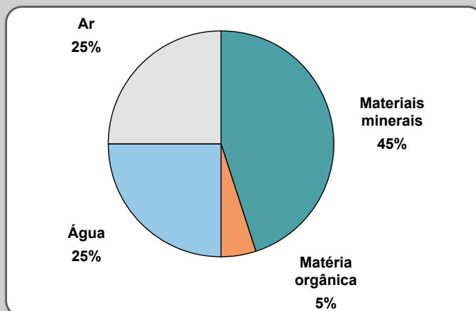
Figura 24 – Esquema da composição do horizonte A de um solo quando em boas condições para crescimento das plantas.
