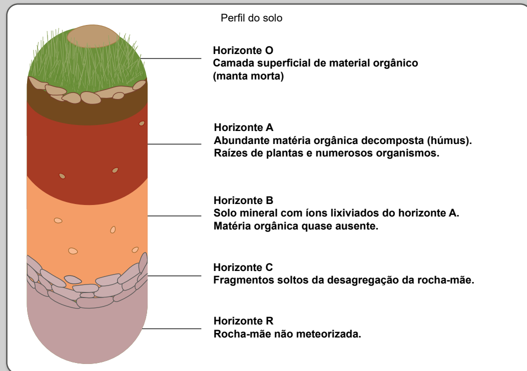
Figura 9 – Esquema de um perfil de solo.
