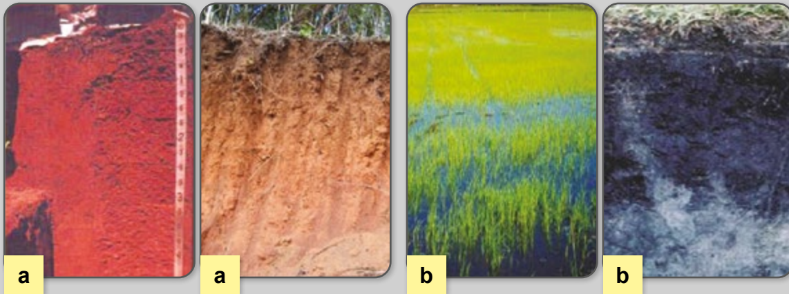
Figura 14 – Solos com boa drenagem (a) e solos mal drenados (b).
