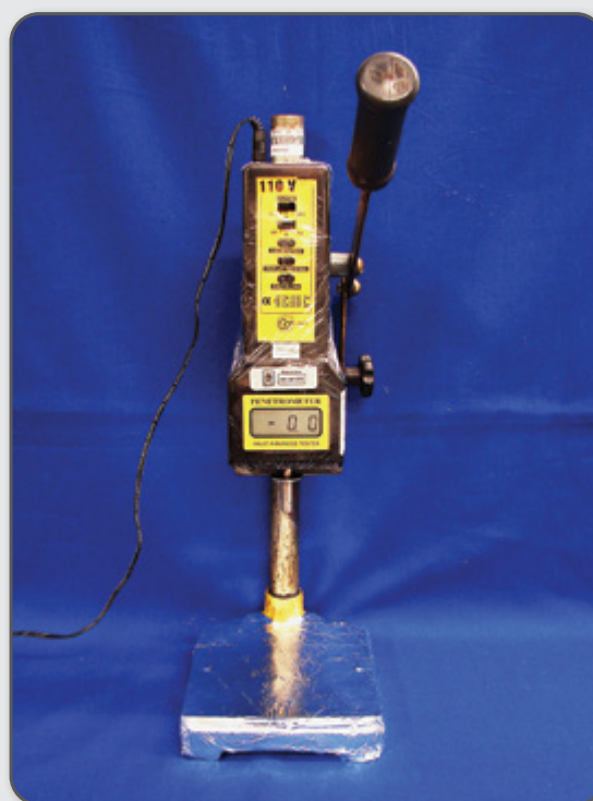
Figura 5 – Penetrômetro digital.
