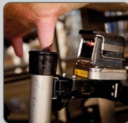
Figura 15 – Vista de um sistema robotizado de ordenha em funcionamento.
