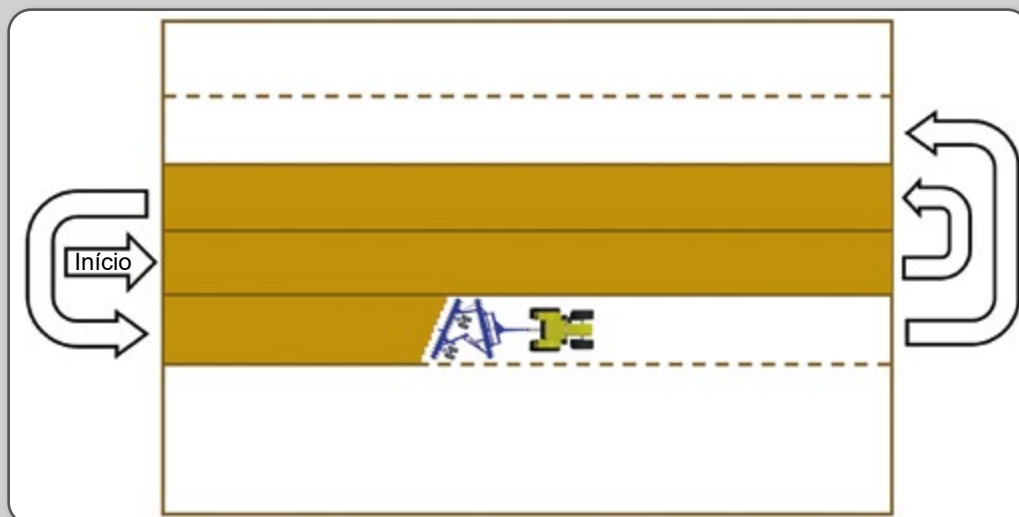
Figura 101 – Gradagem de dentro para fora em talhão retangular.
