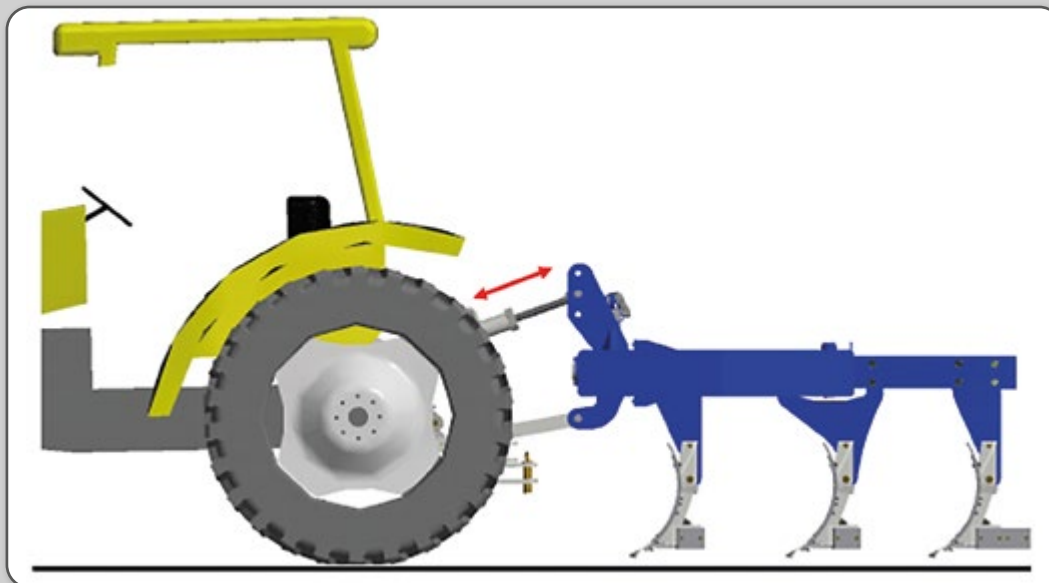
Figura 50 – Nivelamento longitudinal.
