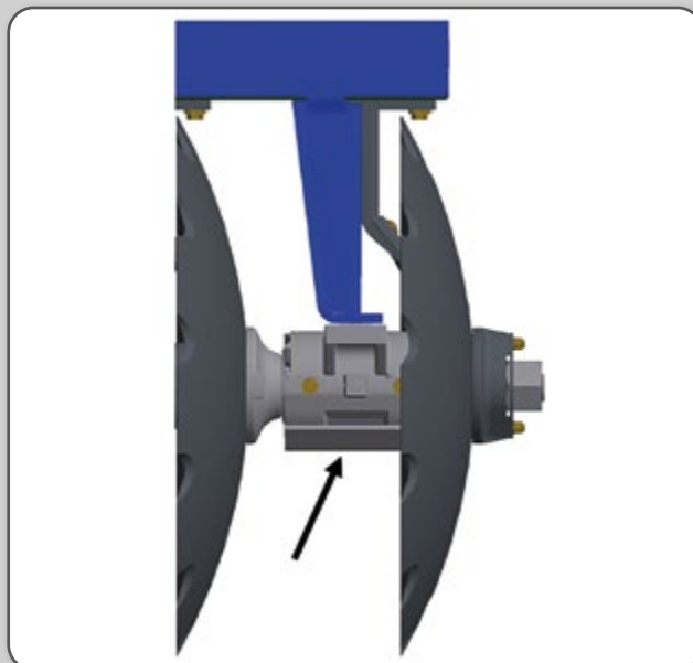
Figura 84 – Detalhe do mancal da grade entre os discos.
