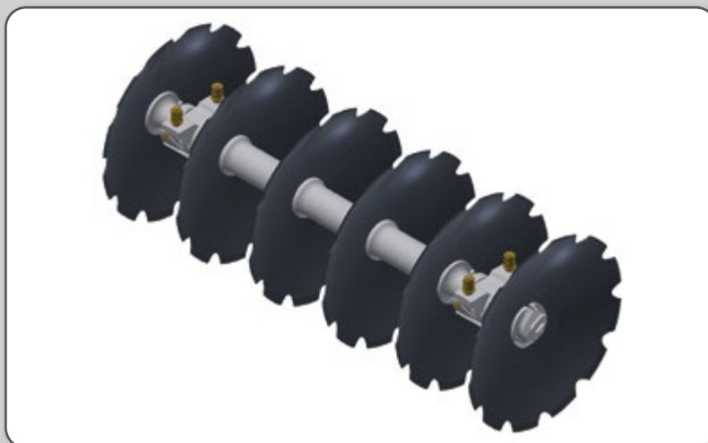
Figura 86 – Representação de uma seção de discos recortados.
