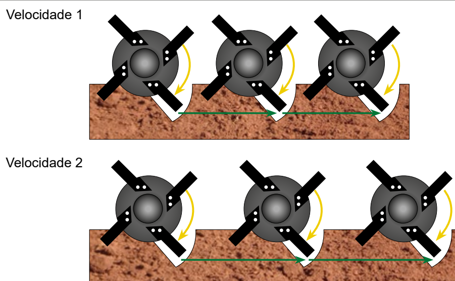
Figura 54 – Aumento da velocidade de deslocamento para uma mesma rotação do rotor.
